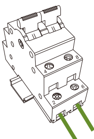
1 Bottom wiring
